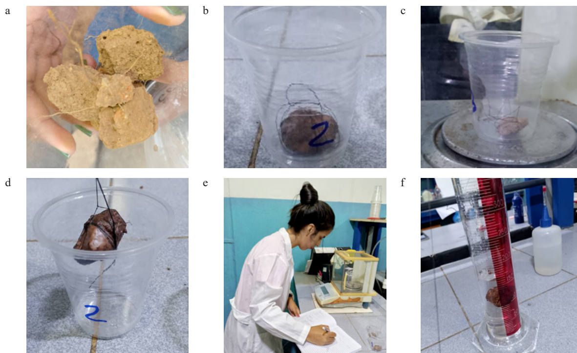
Figura 5. Densidad aparente ( \rho_A ) mediante el método de la parafina, a) agregado de suelo (no disturbado y seco), b) agregado de suelo atado a un hilo, c) pesada del conjunto ( P_{ss} ). d) recubrimiento del agregado en parafina, e) pesada del conjunto ( P_{sp} ) y e) determinación del volumen del agregado parafinado ( V_a )
