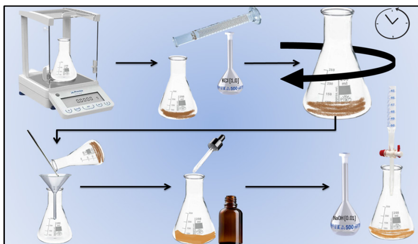
Figura 9. Diagrama del procedimiento de acidez intercambiable del suelo (7)
