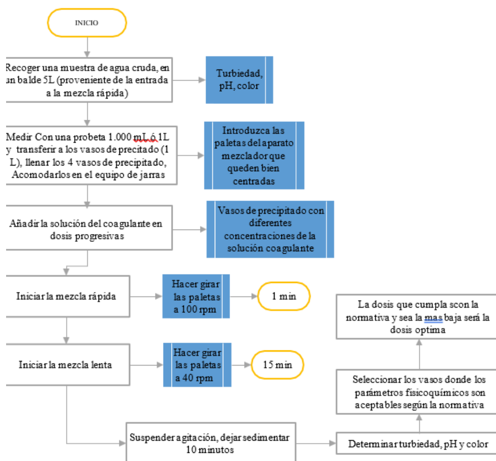
Figura 20. Metodología para la Obtención de la Dosis Optima de Coagulante
