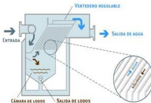
Figura 9. Partes que Conforman un Sedimentador Laminar (13)
