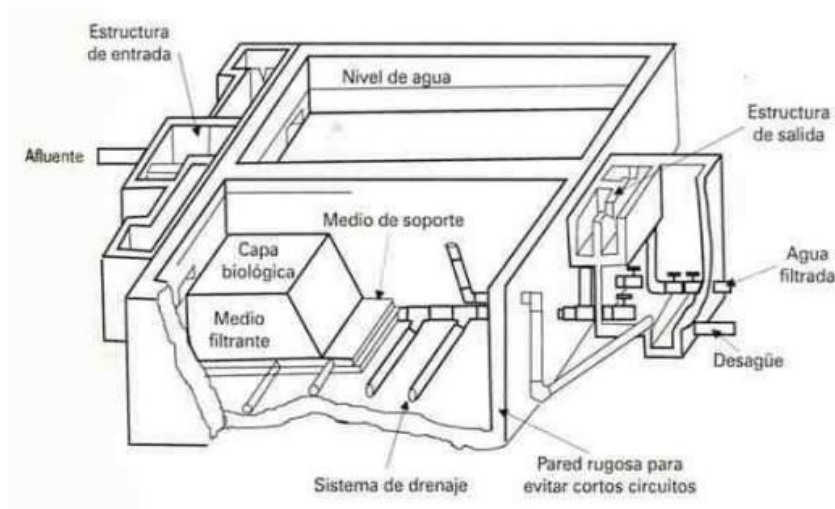
Figura 19. Componentes de Filtro lento (15)
