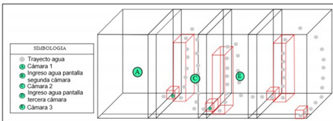
Figura 18. Trayecto del Agua en las 4 Primeras Cámaras del Floculador (12)
