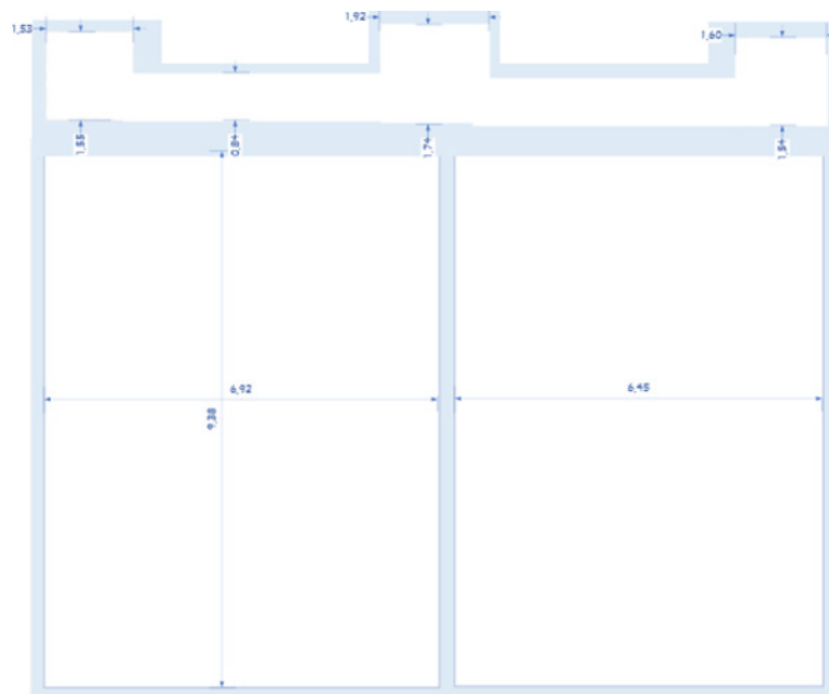
Figura 13. Estructura Filtro Lento y Dimensiones
