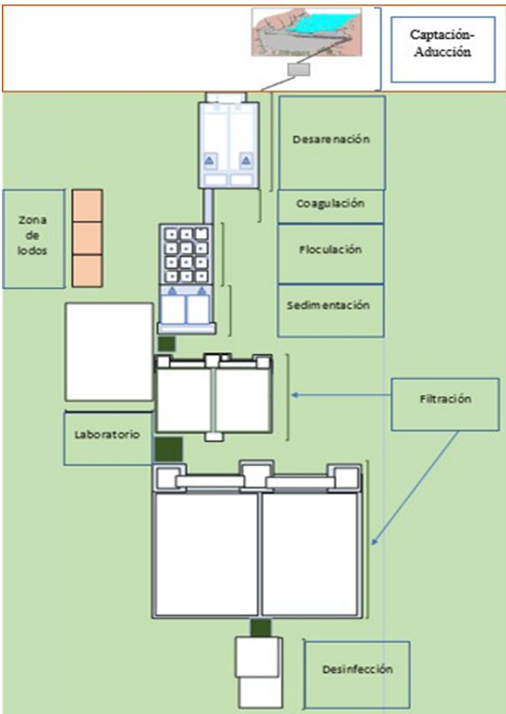
Figura 1. Layout PTAP Topacio
