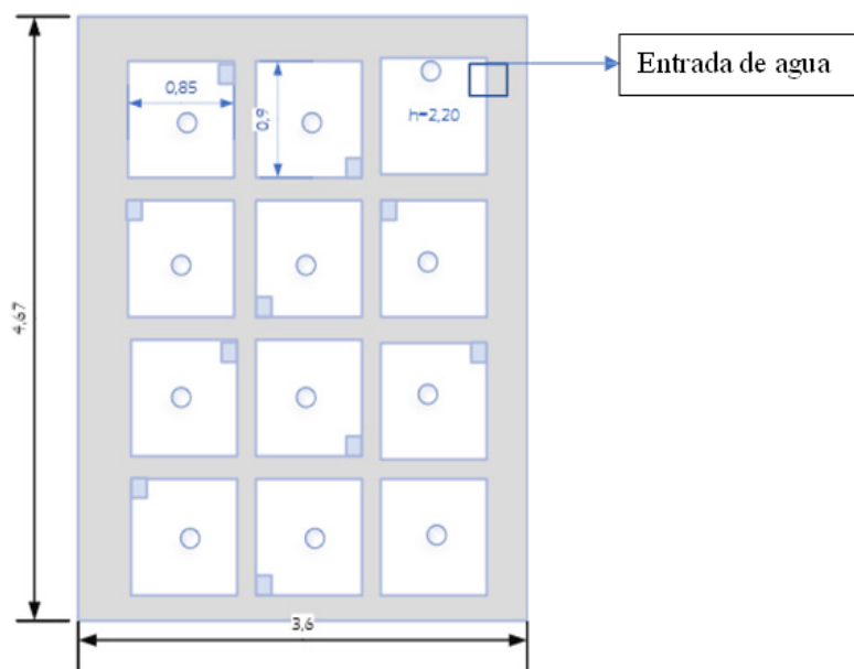
Figura 7. Esquema Floculador Tipo Alabama
