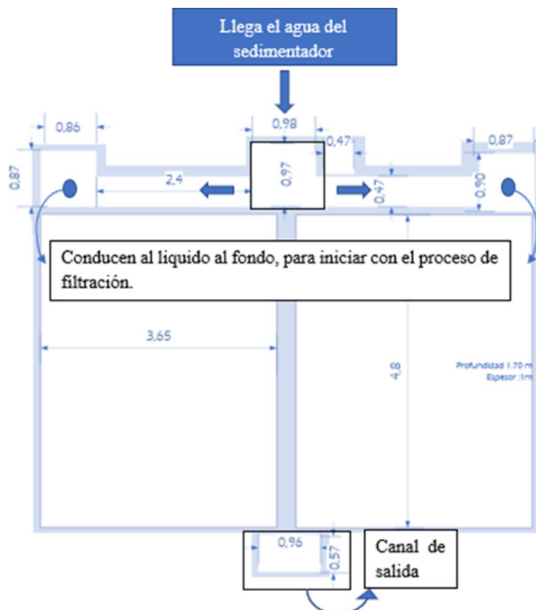
Figura 12. Filtro Rápido con Dimensiones
