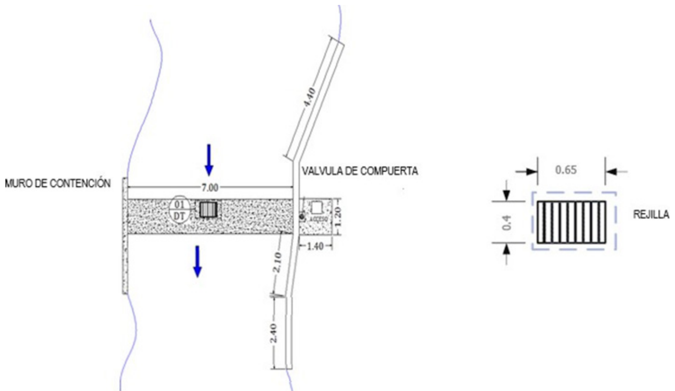
Figura 3. Esquema de Captación-Bocatoma de Fondo (4)
