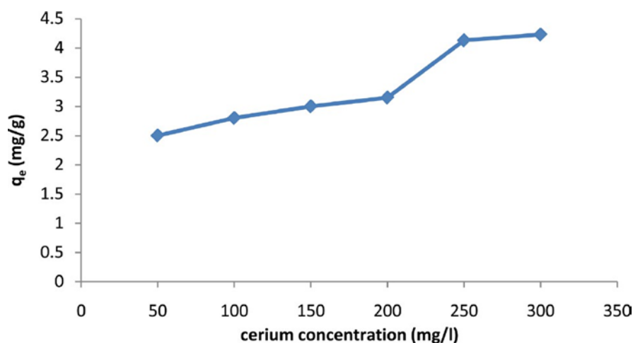
Figura 7. Efectos de la concentración inicial de iones de cerio sobre la adsorción de cerio por el carbón activado (35)
