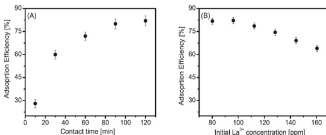
Figura 5. Eficiencia de adsorción vs A) tiempo de contacto, B) concentración inicial (33)
