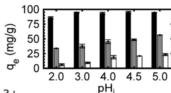
Figura 9. Dependencia del pH con la adsorción de Eu
