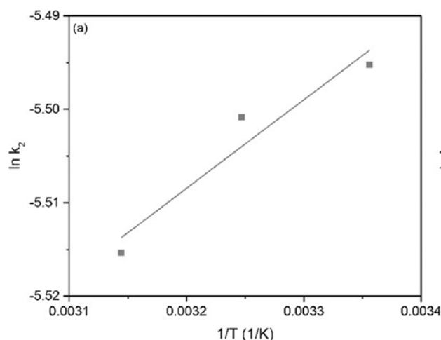
Figura 13. Gráfico de Arrhenius para la adsorción de Eu por celulosa funcionalizada
