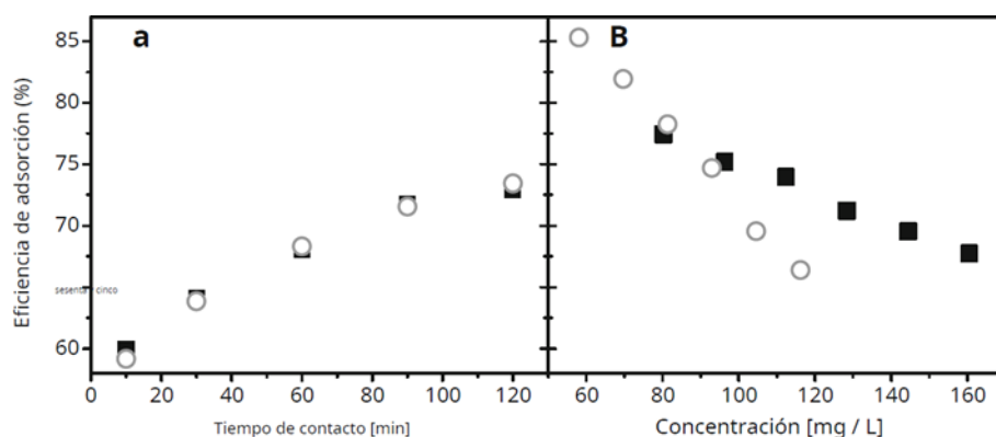
Figura 4. El recuadro negro hace referencia al ion La, a) eficiencia de adsorción vs tiempo de contacto, b) eficiencia de adsorción vs concentración inicial (31)
