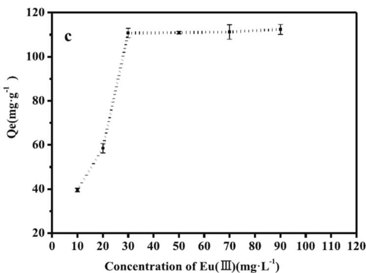
Figura 11. Concentración inicial de Eu vs la capacidad de adsorción (39)
