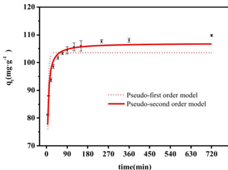
Figura 10. Análisis cinético adsorción de Eu con Serratia marcescens (39)
