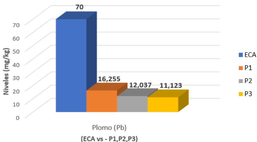
Figura 18. Resultados de las concentraciones de Plomo (Pb) con el ECA
