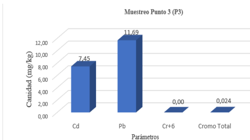
Figura 15. Resultado de ensayo de Metales pesados, punto 3
