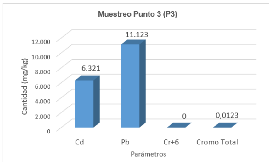
Figura 8. Resultado de ensayo de Metales pesados, punto 3
