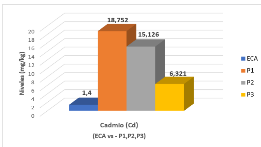
Figura 10. Resultados de las concentraciones de Cadmio (Cd) con el ECA
