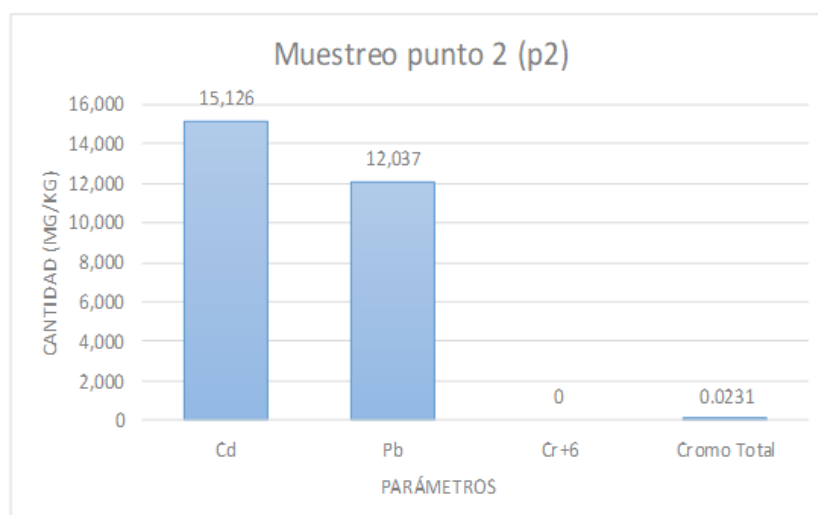
Figura 7. Resultado de ensayo de Metales pesados, punto 2
