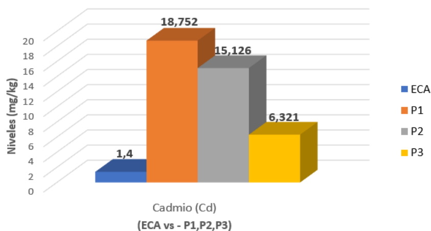
Figura 17. Resultados de las concentraciones de Cadmio (Cd) con el ECA
