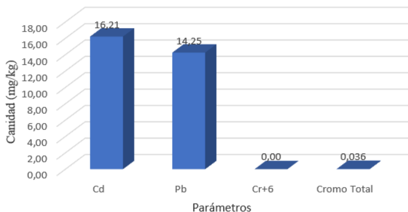
Figura 14. Resultado de ensayo de Metales pesados, punto 2
