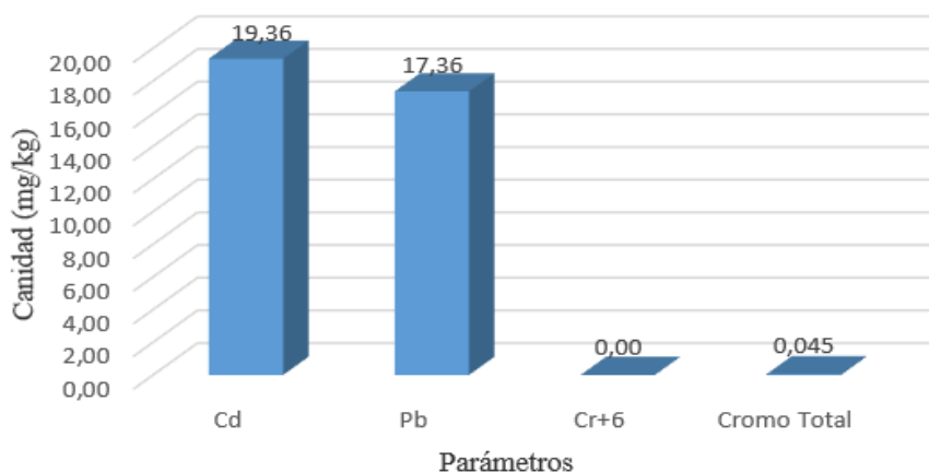
Figura 13. Resultado de ensayo de Metales pesados, punto 1
