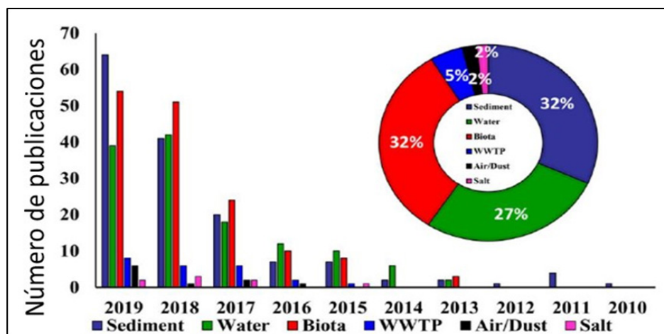
Figura 5. Resultados de literatura usando FTIR
