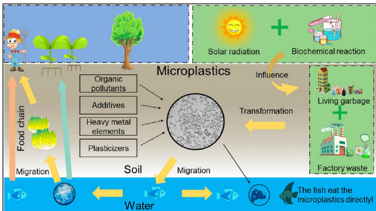
Figura 3. El origen, la migración y los daños de los microplásticos
